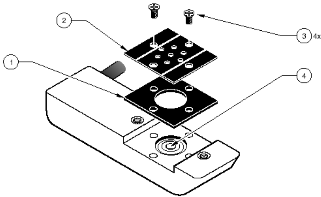
图 47 移开保护盖
